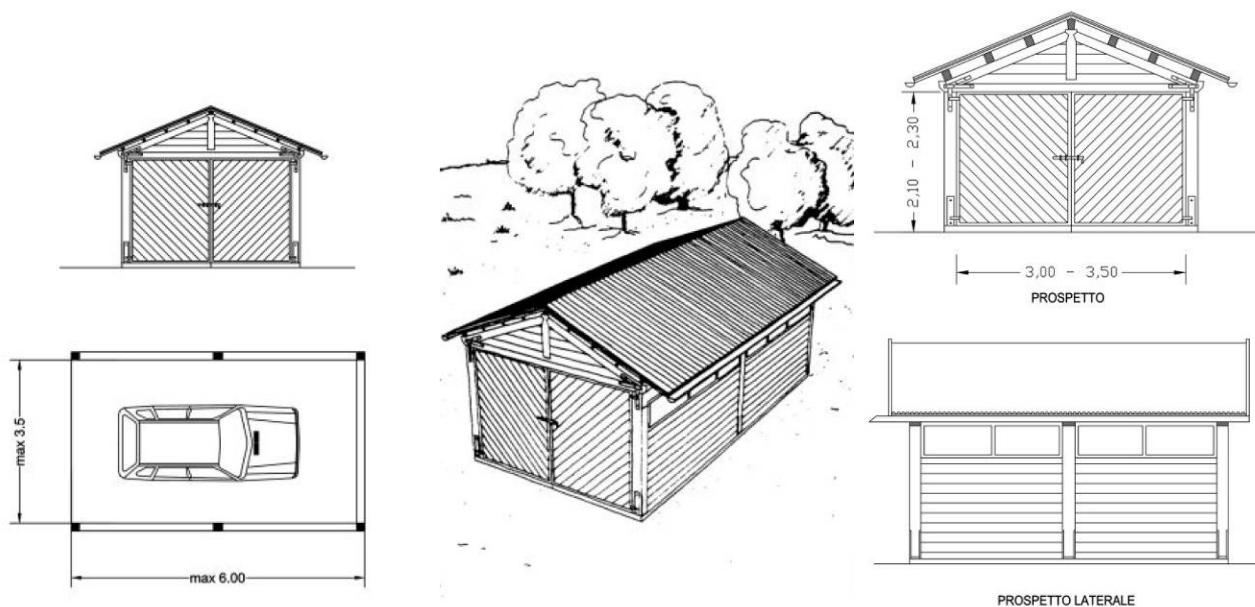
Schemi dimensionali di locali accessori ad uso autorimessa
