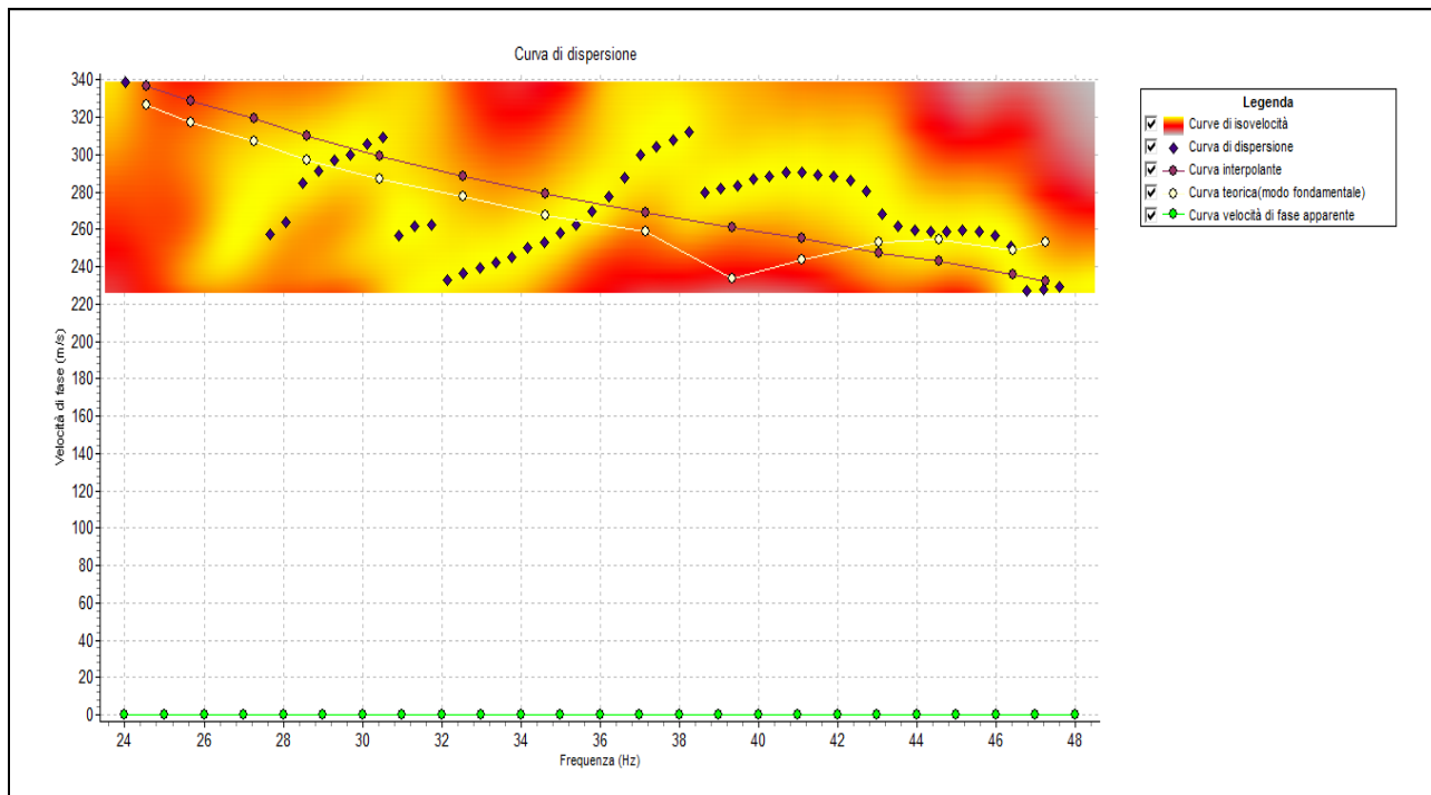
Figura 3: Curva di dispersione
