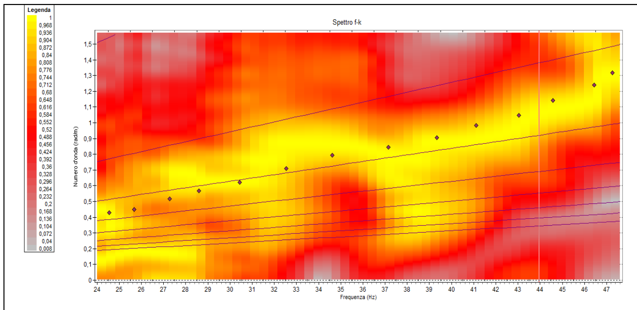
Figura 2: Spettro f - k
