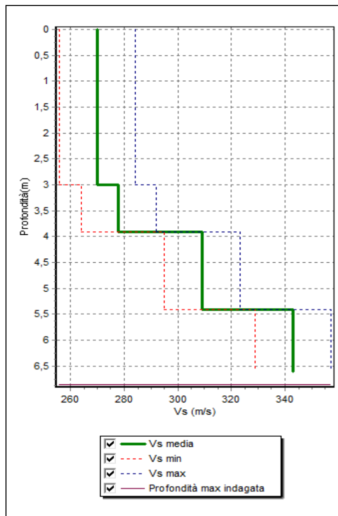
Figura 4: Profilo Vs numerico
