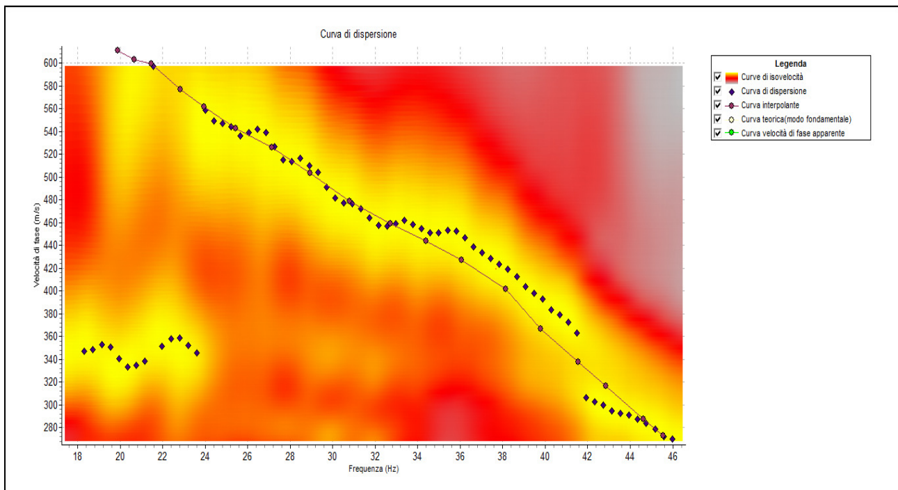
Figura 3: Curva di dispersione
