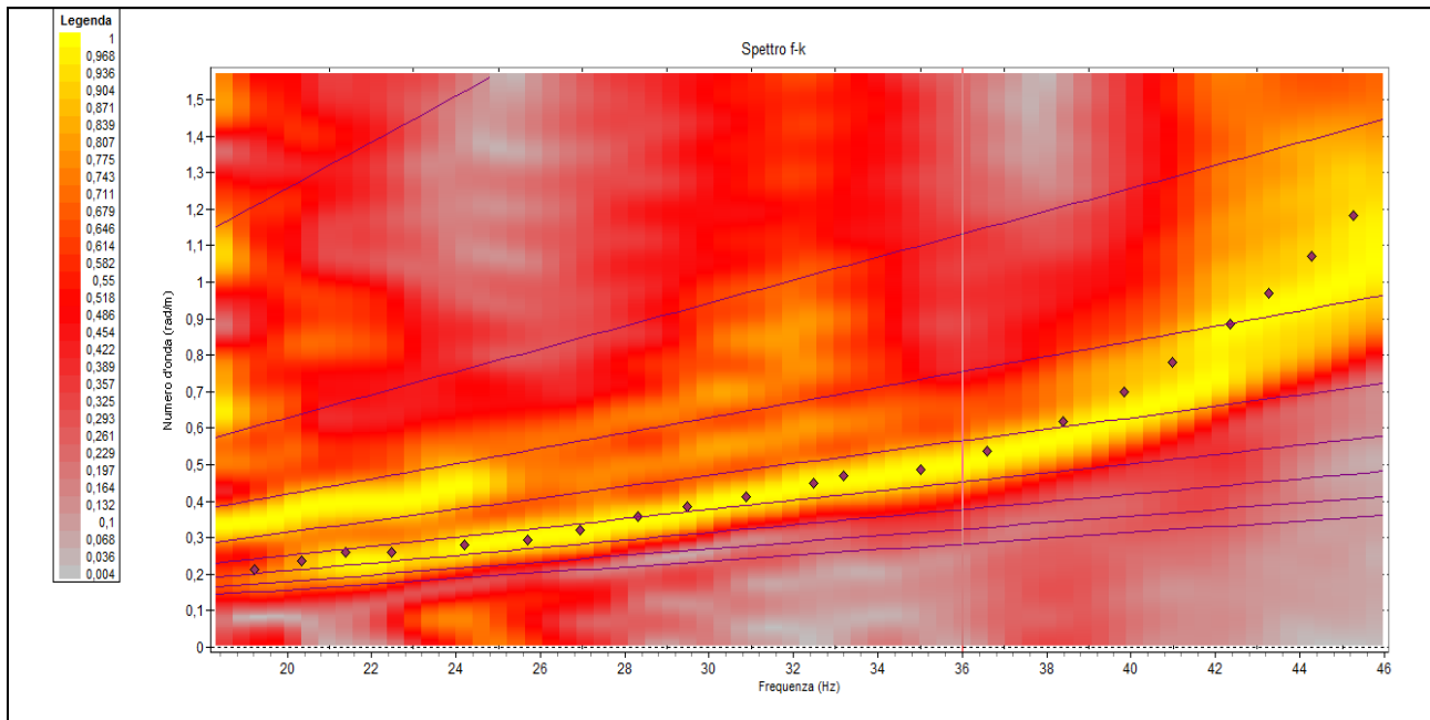
Figura 2: Spettro f - k
