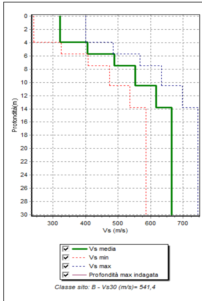
Figura 4: Profilo Vs numerico
