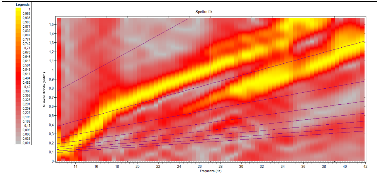
Figura 2: Spettro f - k
