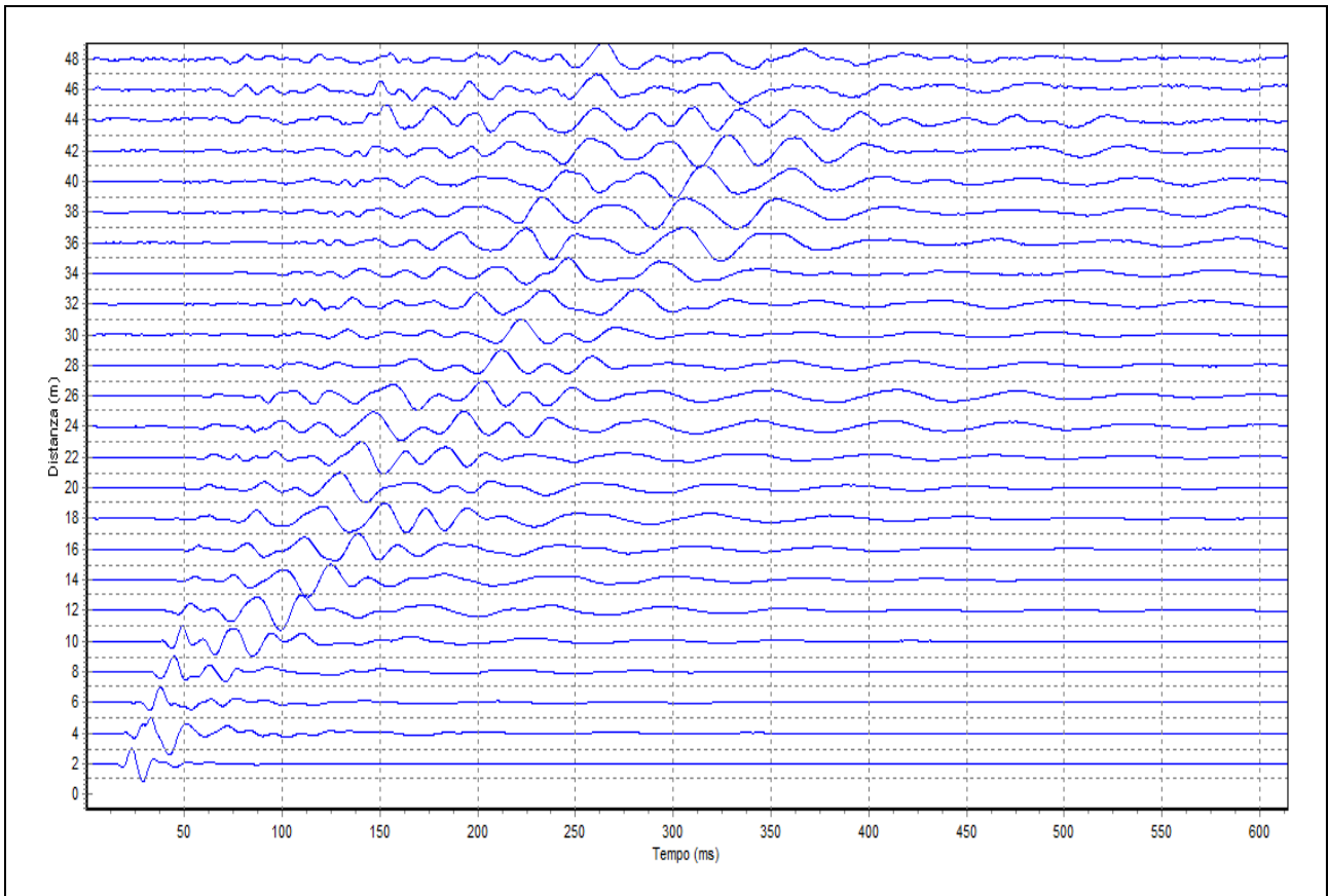
Figura 1: Tracce sperimentali
