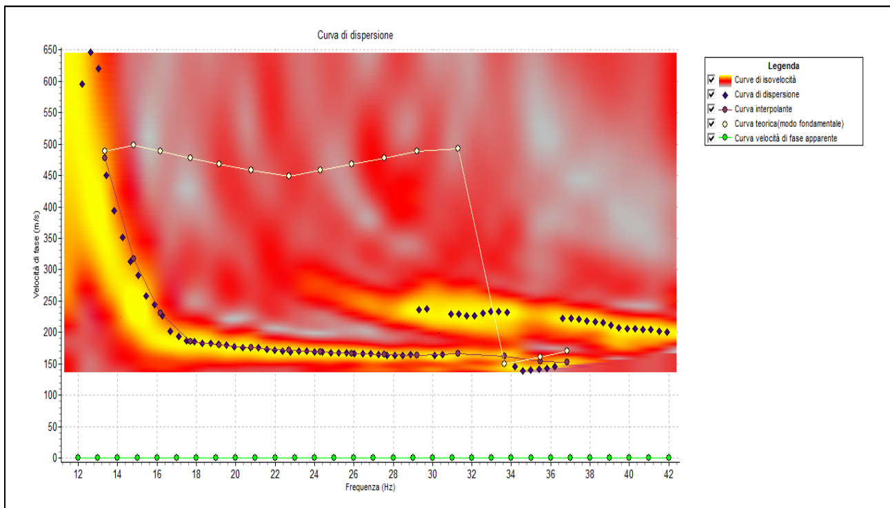
Figura 3: Curva di dispersione
