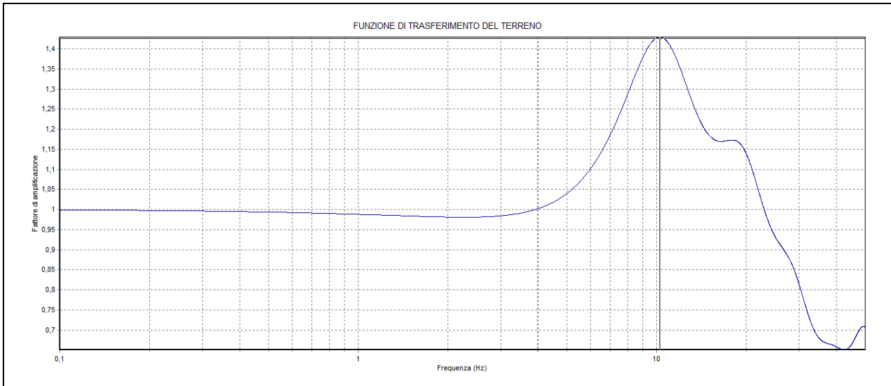
Figura 5: Funzione di trasferimento
